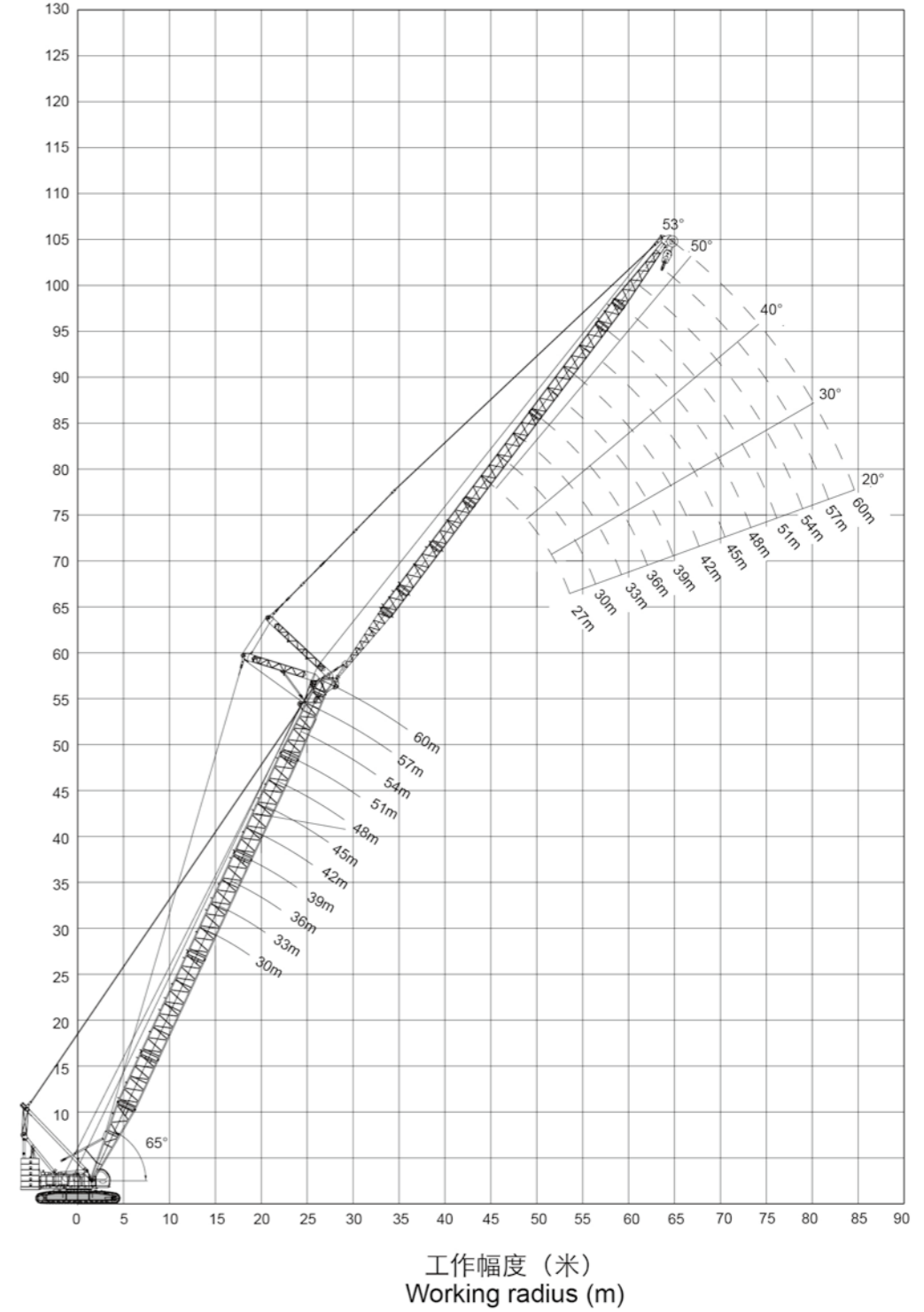
主臂65°时 Boom angle at 65°
