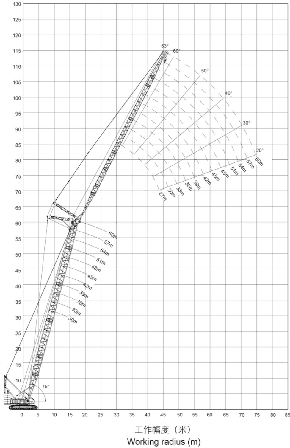
主臂75°时 Boom angle at 75°
